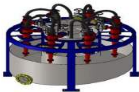
هیدروسیکلون ۶ خوشه‌ای طراحی شده برای کارخانه ۲
