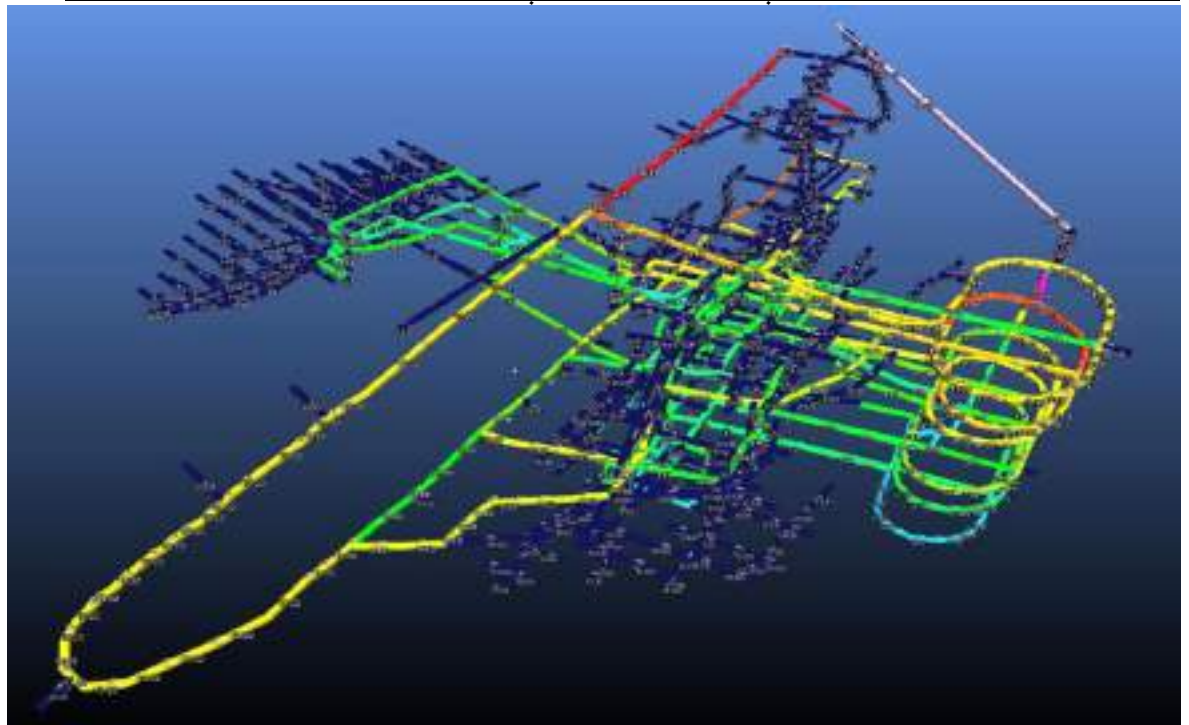
طراحی سیستم تهویه زون ۱ و غرب گوشفیل
